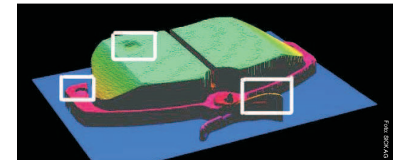
Kontrolle von Bremsbelägen
