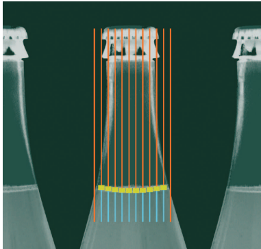
Füllstandsmessung
